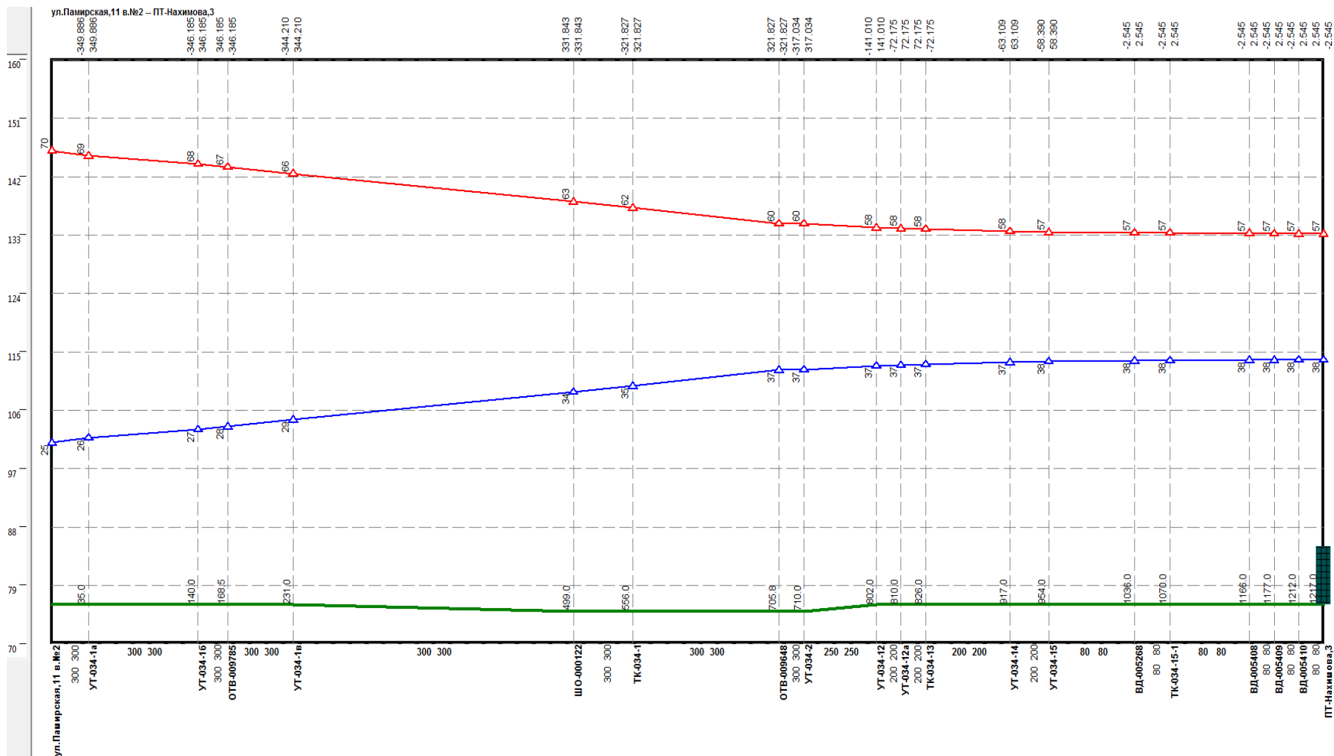
Рисунок 2.16 –Результат гидравлического расчета - график гидравлических режимов по пути теплоносителя от ТЭЦ-3 до ПТ-Нахимова,3
