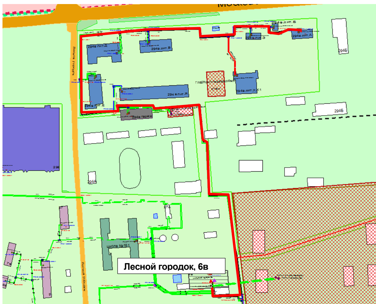
Рисунок 2.19 – Результат гидравлического расчета - расчетный путь теплоносителя от Лесной городок 6в до ПТ-Моск.ш,294в лит.А
