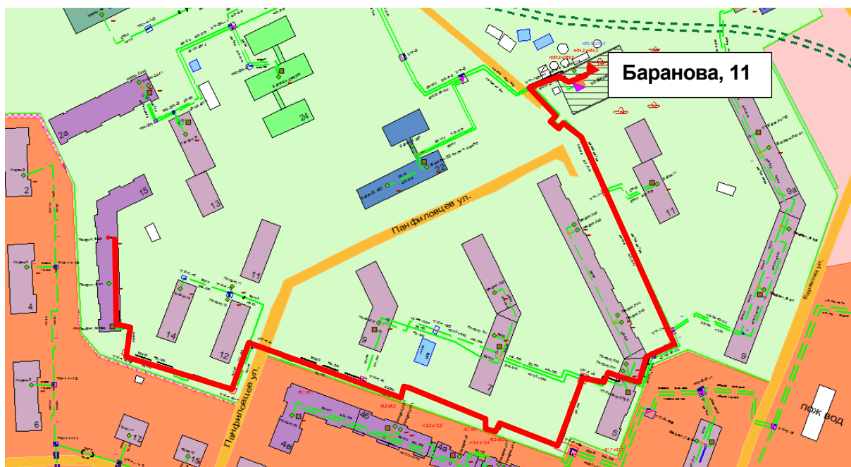
Рисунок 2.41 – Результат гидравлического расчета - расчетный путь теплоносителя от котельной Баранова, 11 до ПТ-Панфил,15 э2
