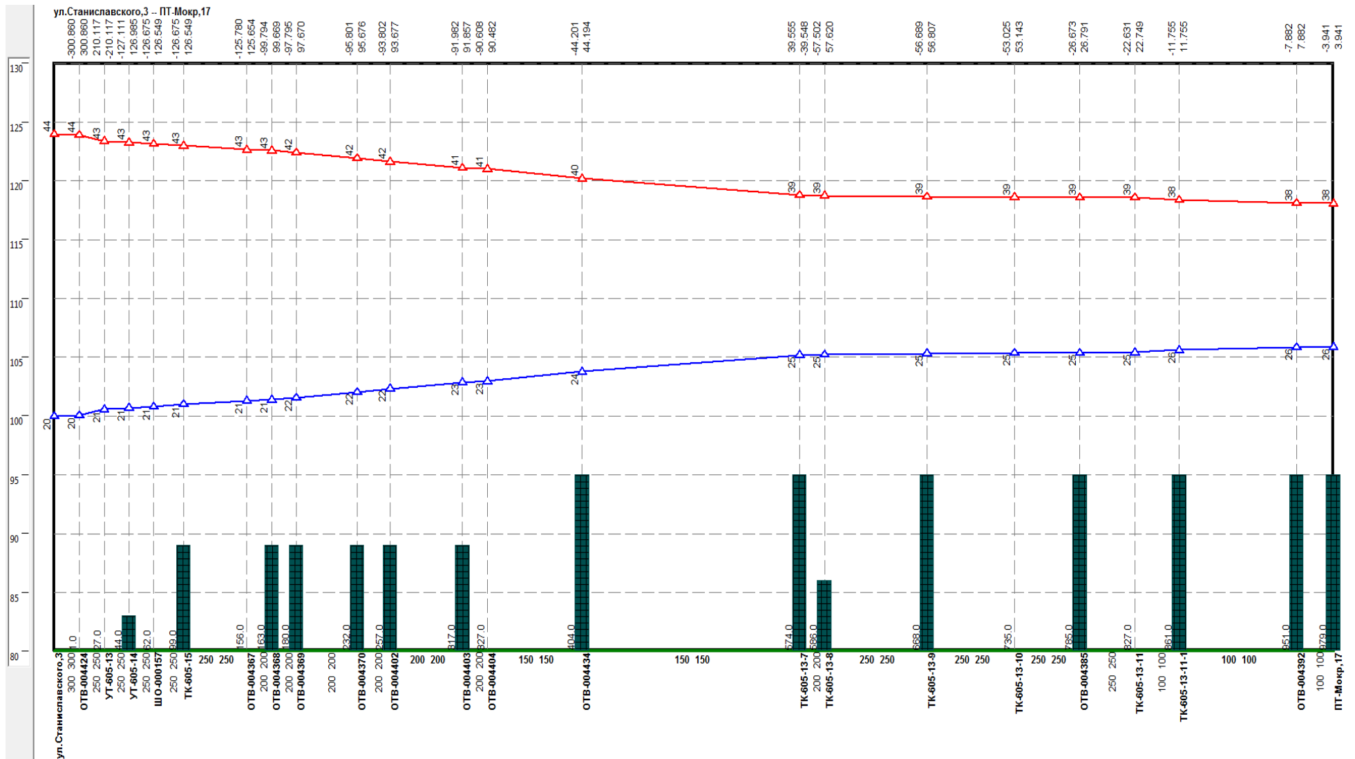
Рисунок 2.50 –Результат гидравлического расчета - график гидравлических режимов по пути теплоносителя от котельной Станиславского, 3 до ПТ-Мокр, 17
