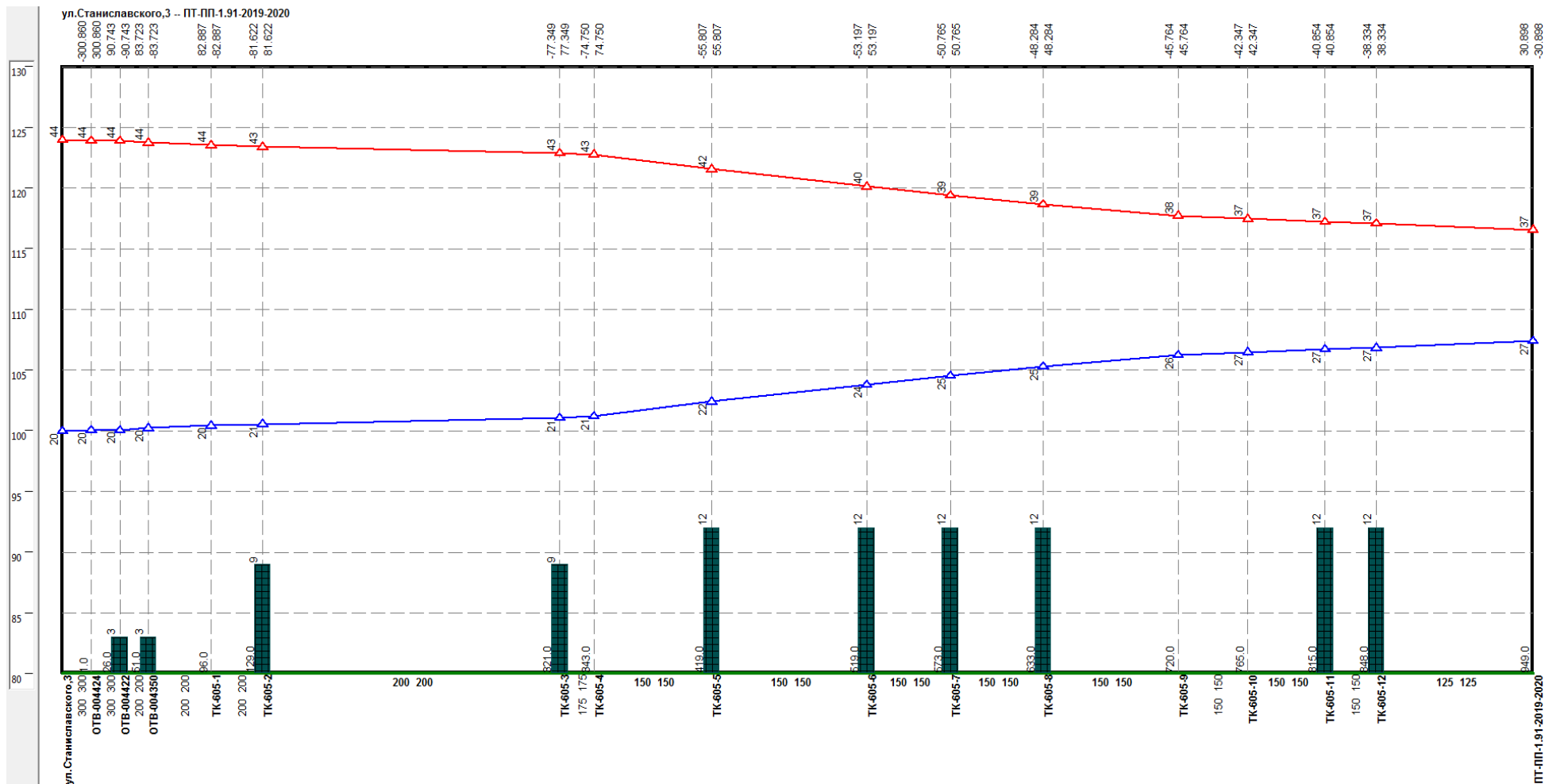
Рисунок 2.48 –Результат гидравлического расчета - график гидравлических режимов по пути теплоносителя от котельной Станиславского, 3 до ПТ- ПП-1,91-2019-2020.
