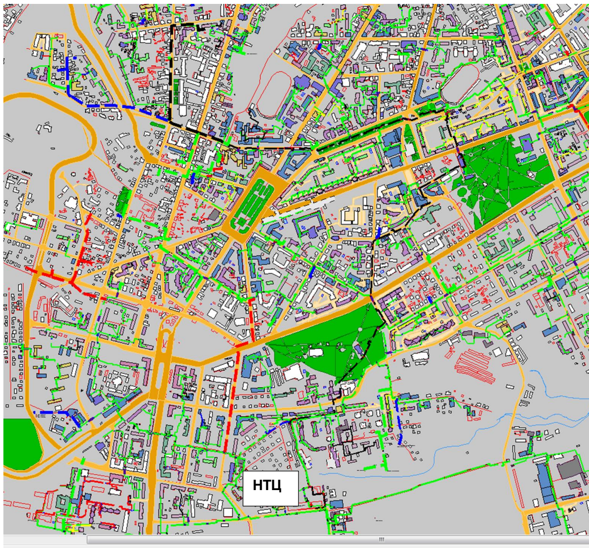
Рисунок 2.63 – Результат гидравлического расчета - расчетный путь теплоносителя от котельной НТЦ до ПТ-ПП-2.161-2017
