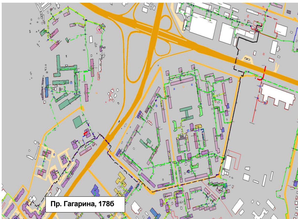
Рисунок 2.69 – Результат гидравлического расчета - расчетный путь теплоносителя от котельной пр. Гагарина, 1786 до ПТ-Гагар.пр.101/5 ИТП №2.
