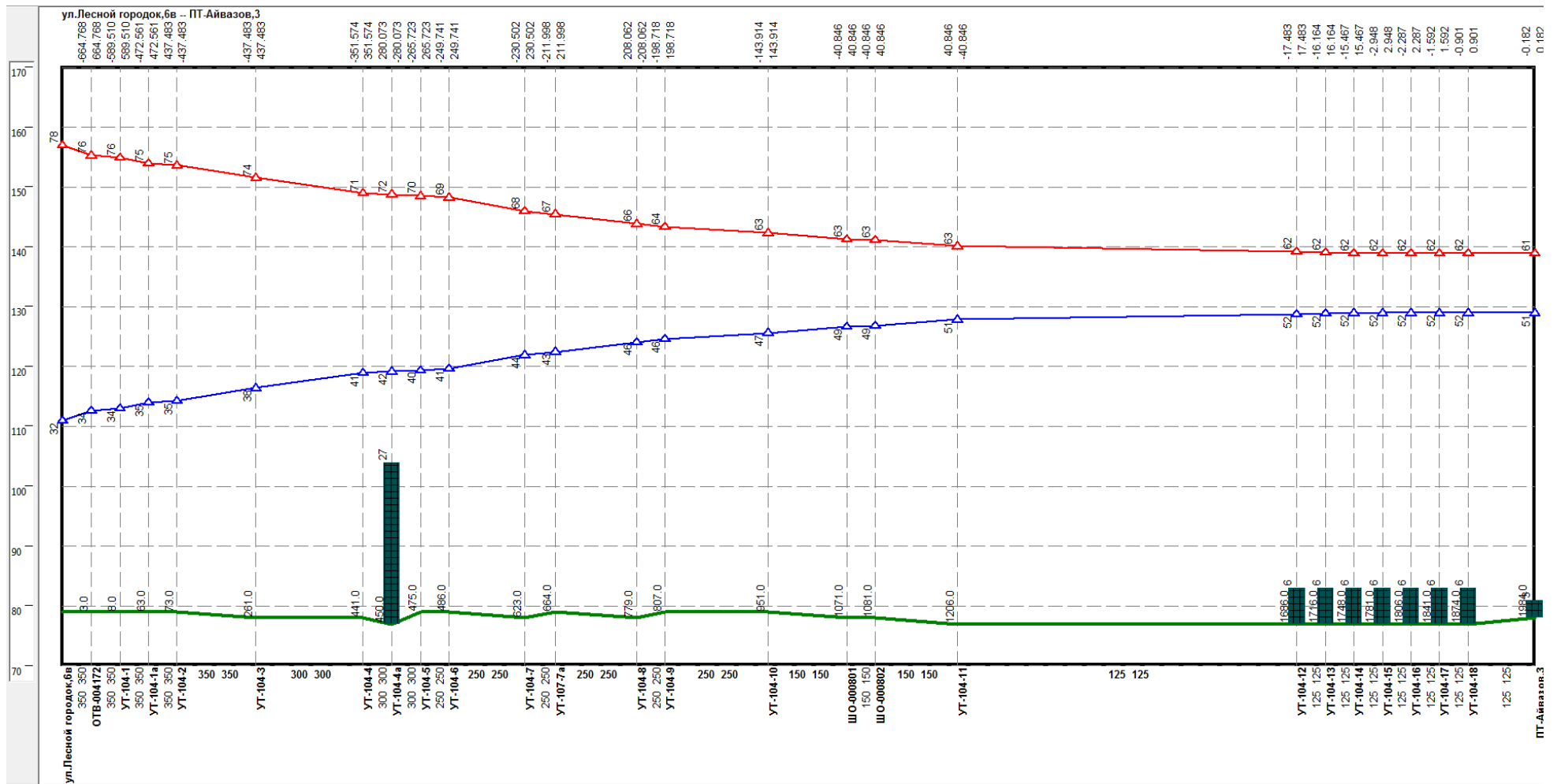
Рисунок 2.18 –Результат гидравлического расчета - график гидравлических режимов по пути теплоносителя от Лесной городок, 6б до ПТ-Айвазов,3
