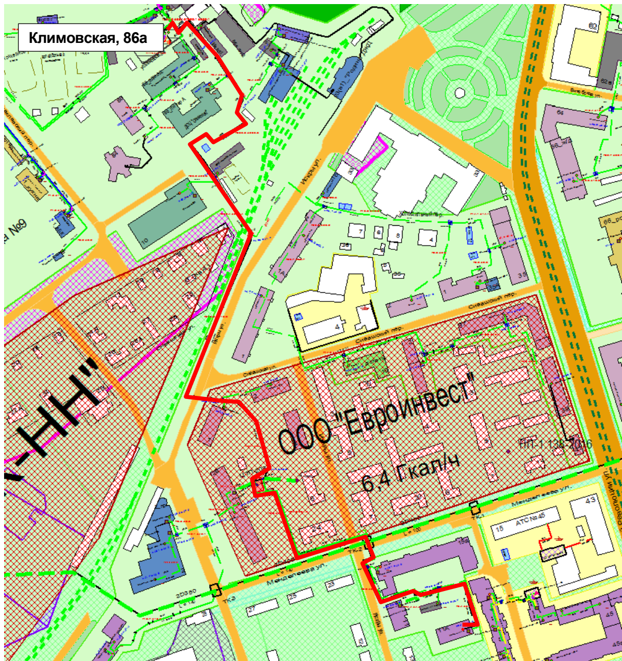
Рисунок 2.43 – Результат гидравлического расчета - расчетный путь теплоносителя от котельной Климовская, 86а до ПТ-Искры,11а
