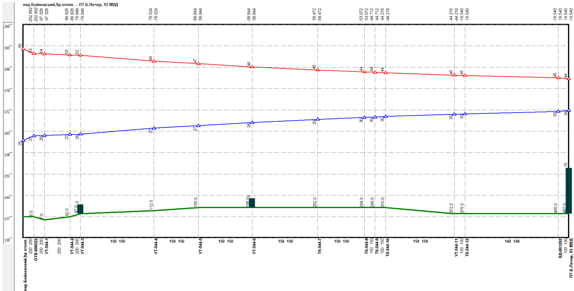
Рисунок 2.24 –Результат гидравлического расчета - график гидравлических режимов по пути теплоносителя от Бойновский, 9д до ПТ-Б.Печер, 93 МВД
