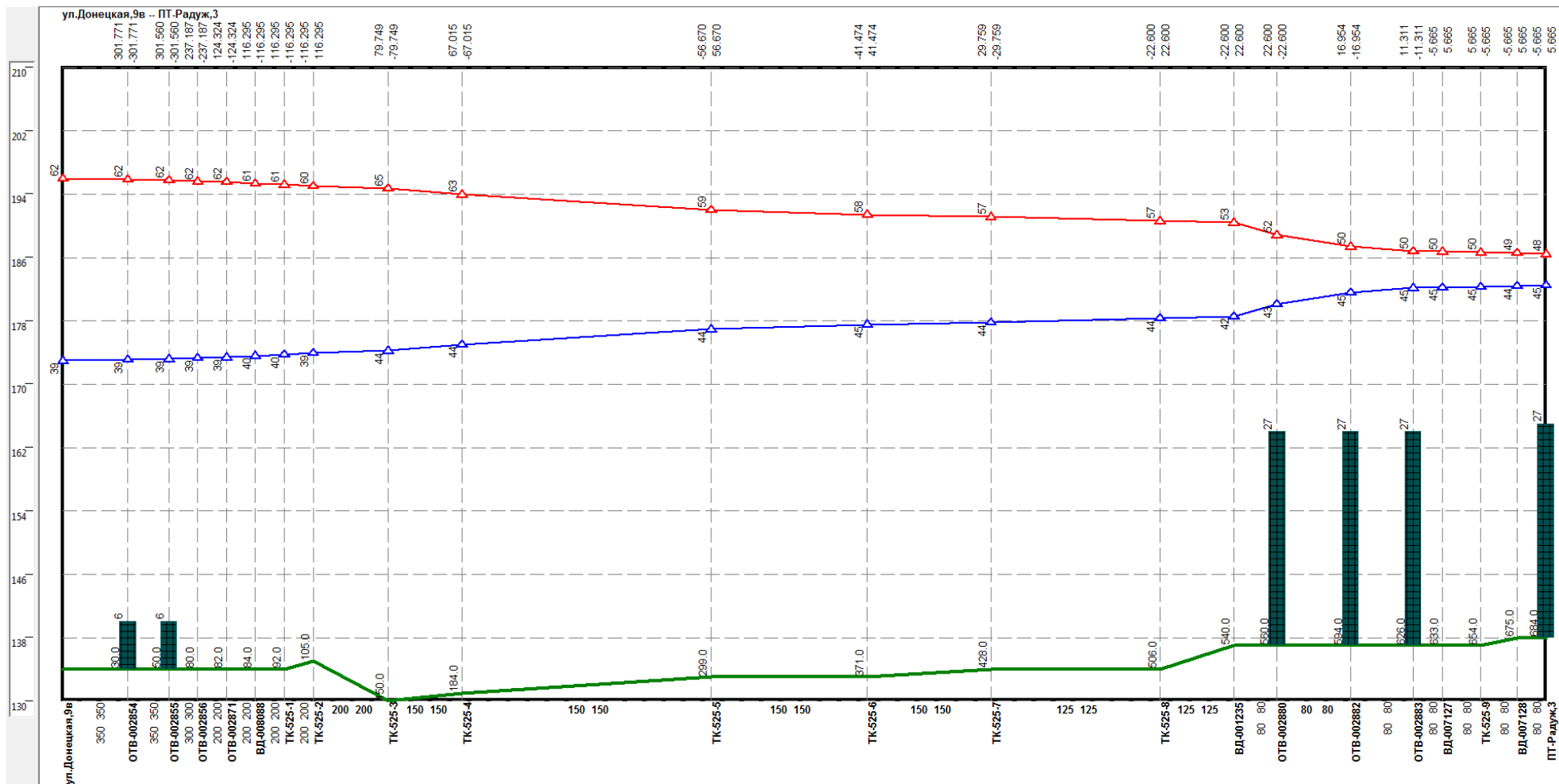
Рисунок 2.72 –Результат гидравлического расчета - график гидравлических режимов по пути теплоносителя от котельной Донецкая, 9-в до ПТ-Радуж,3
