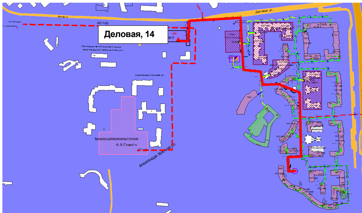
Рисунок 2.27 – Результат гидравлического расчета - расчетный путь теплоносителя от котельной Деловая, 14 до ПТ-Род.199/2_н
