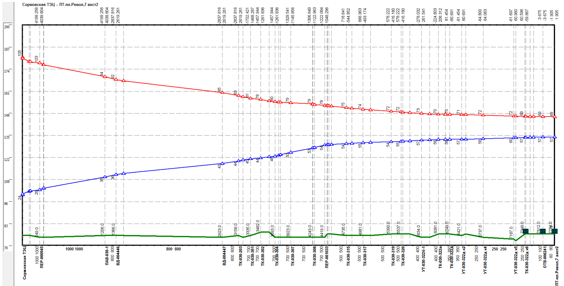
Рисунок 2.6 –Результат гидравлического расчета - график гидравлических режимов по пути теплоносителя от СТЭЦ до ПТ-пл.Револ,7 вест2.
