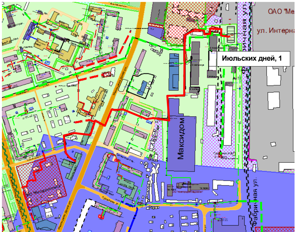
Рисунок 2.31 – Результат гидравлического расчета - расчетный путь теплоносителя от Июльских дней, 1 до ПТ-Июльские дни, 10 школа
