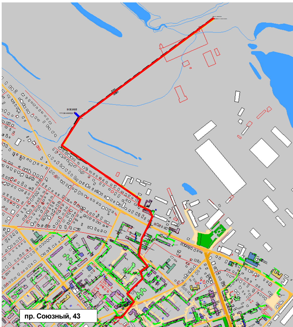
Рисунок 2.73 – Результат гидравлического расчета - расчетный путь теплоносителя от котельной пр. Союзный, 43 до ПТ-ПП-4.101/1.182-2018/2027
