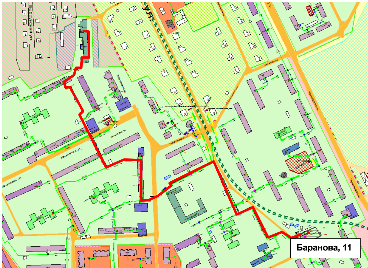
Рисунок 2.39 – Результат гидравлического расчета - расчетный путь теплоносителя от котельной Баранова, 11 до ПТ-Мечн,74 маст
