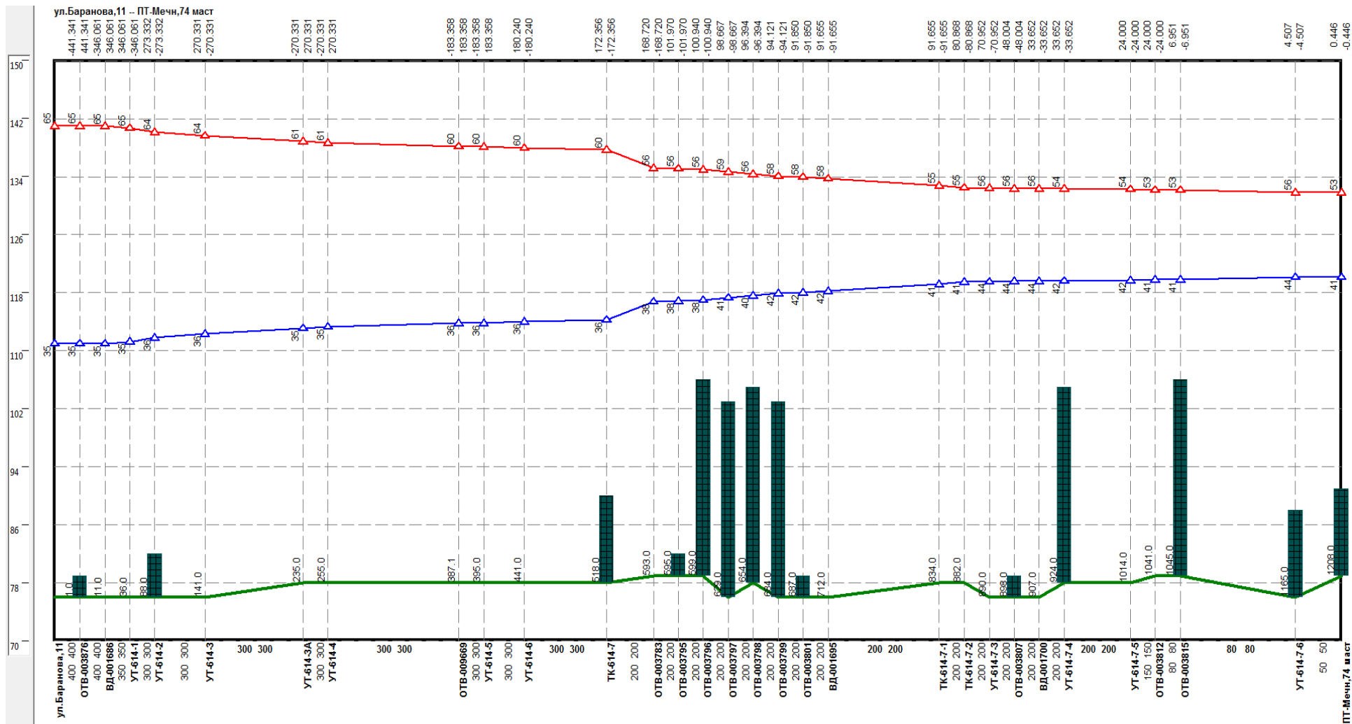
Рисунок 2.40 –Результат гидравлического расчета - график гидравлических режимов по пути теплоносителя от котельной Баранова, 11 до ПТ-Мечн,74 маст
