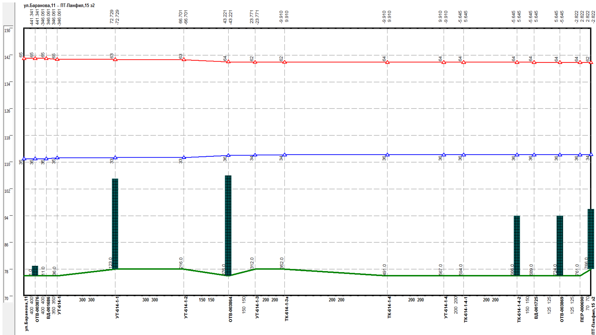
Рисунок 2.42 –Результат гидравлического расчета - график гидравлических режимов по пути теплоносителя от Бойновский, 9д до ПТ-Б.Печер, 93 МВД
