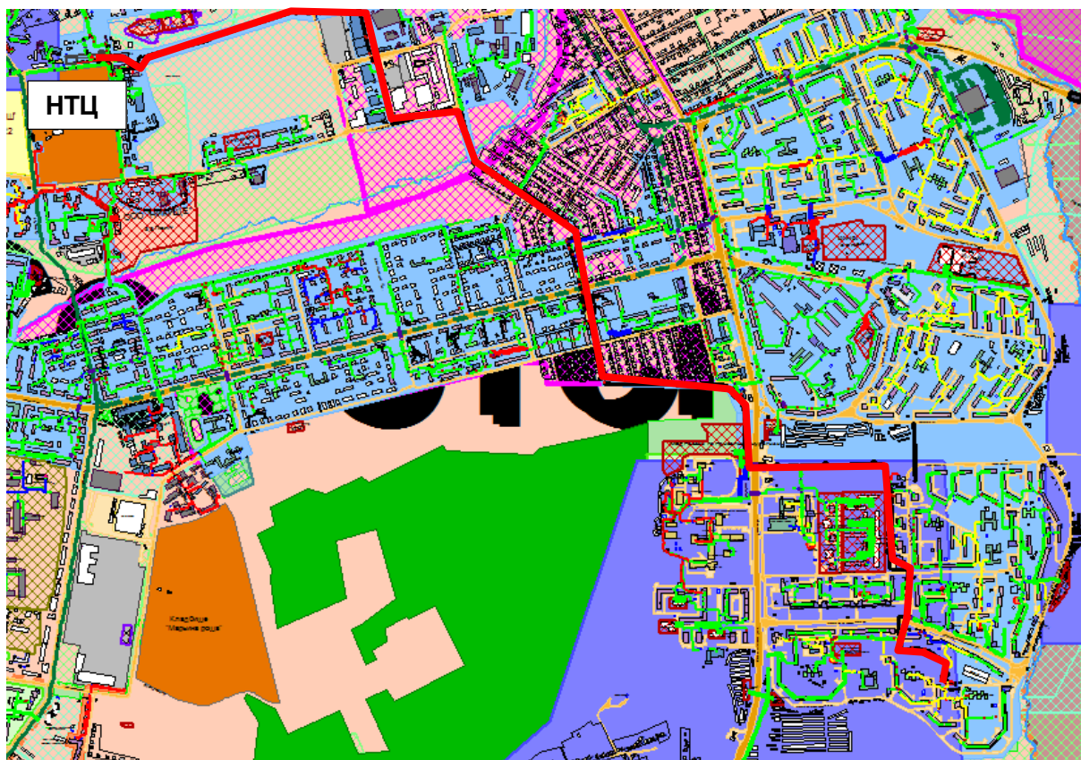
Рисунок 2.59 – Результат гидравлического расчета - расчетный путь теплоносителя от котельной НТЦ до ПТ-Малин,2 пристрой
