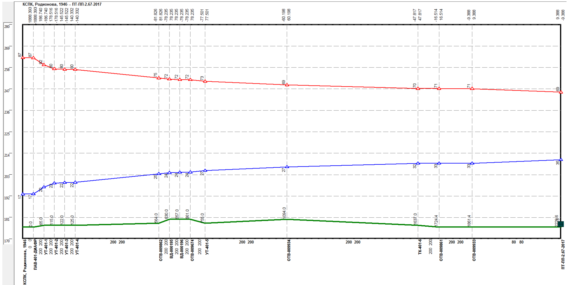
Рисунок 2.78 –Результат гидравлического расчета - график гидравлических режимов по пути теплоносителя от котельной ул. Родионова, 1946 до ПТ-ПП-2.67-2017
