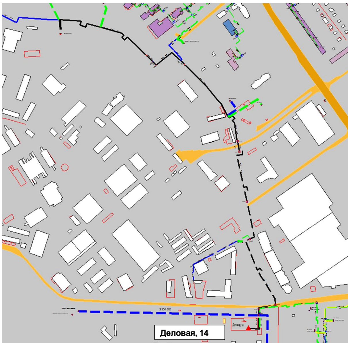
Рисунок 2.29 – Результат гидравлического расчета - расчетный путь теплоносителя от котельной Деловая, 14 до ПТ-ПП-2.99-2017-2018
