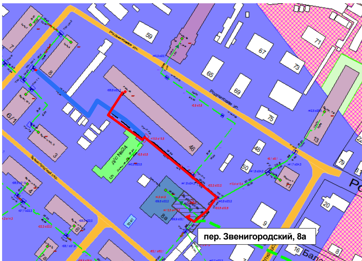
Рисунок 2.53 – Результат гидравлического расчета - расчетный путь теплоносителя от котельной пер. Звенигородский до ПТ-Родн,46
