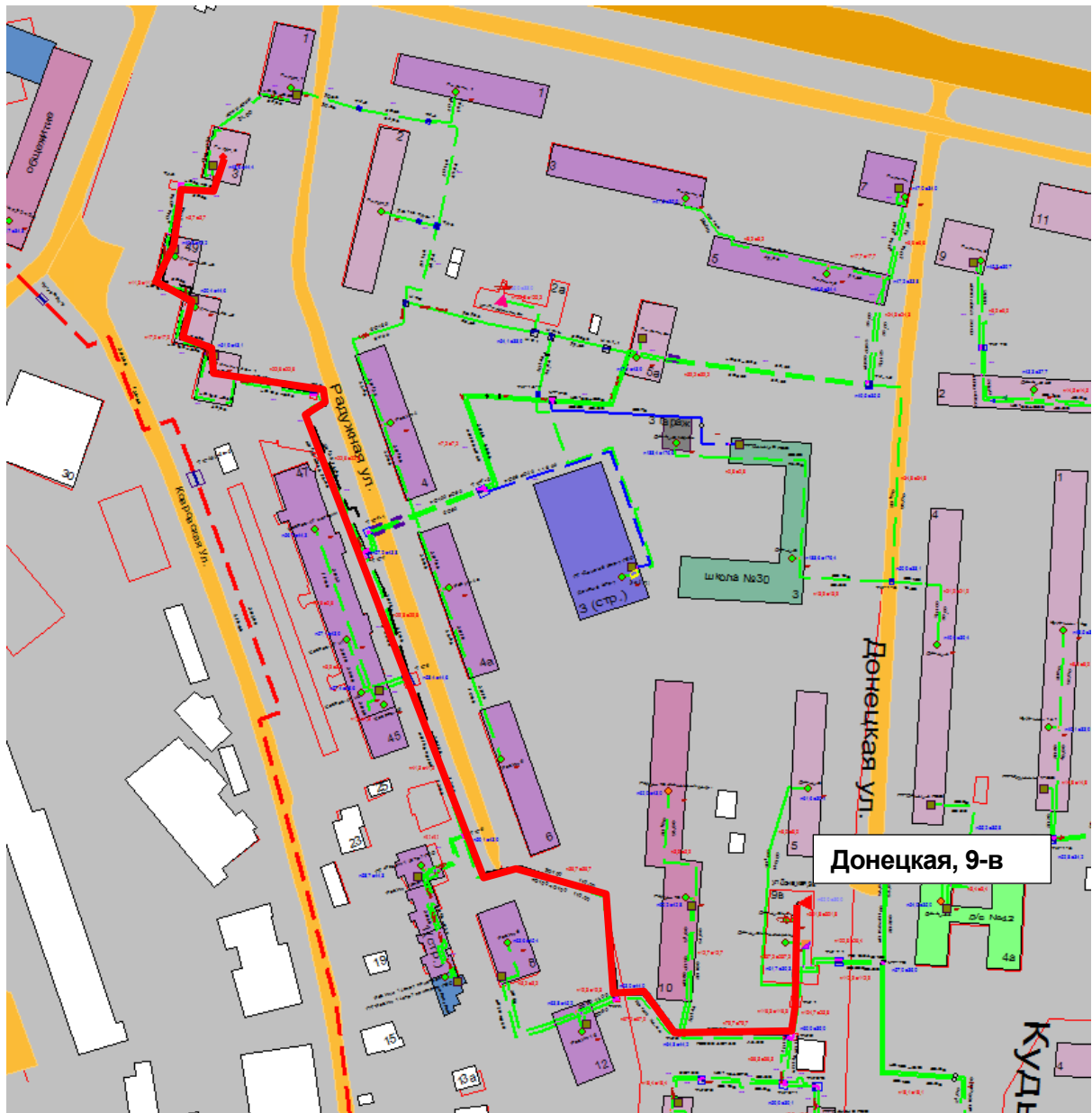
Рисунок 2.71 – Результат гидравлического расчета - расчетный путь теплоносителя от котельной Донецкая, 9-в до ПТ-Радуж,3
