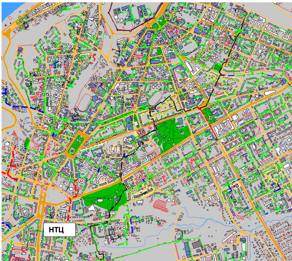
Рисунок 2.61 – Результат гидравлического расчета - расчетный путь теплоносителя от котельной НТЦ до ПТ- ПП-2-50-2015.
