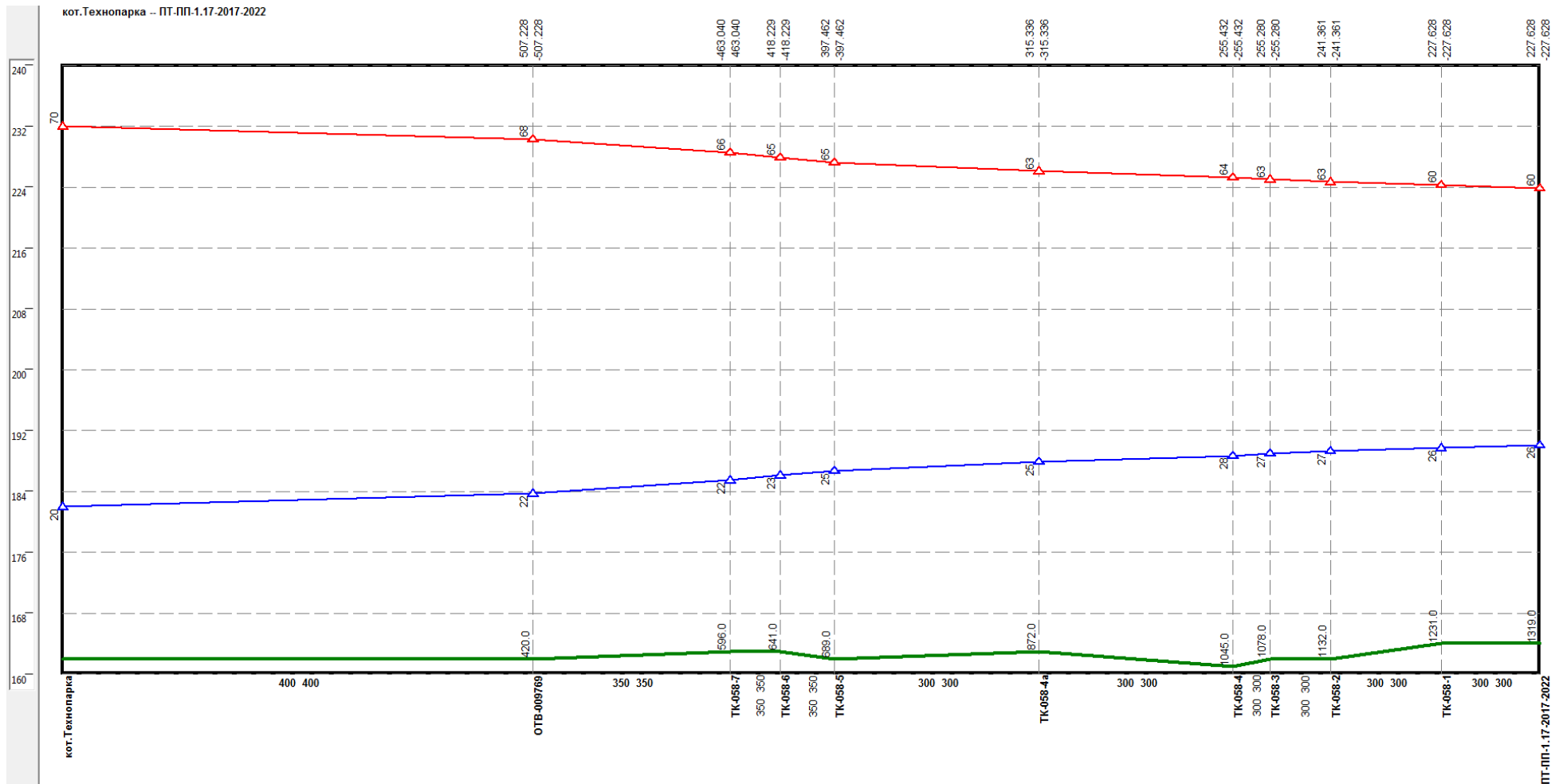
Рисунок 2.36 –Результат гидравлического расчета - график гидравлических режимов по пути теплоносителя 1 от котельной «ТЕХНОПАРК» до ПТ-ПП-2.67-2017
