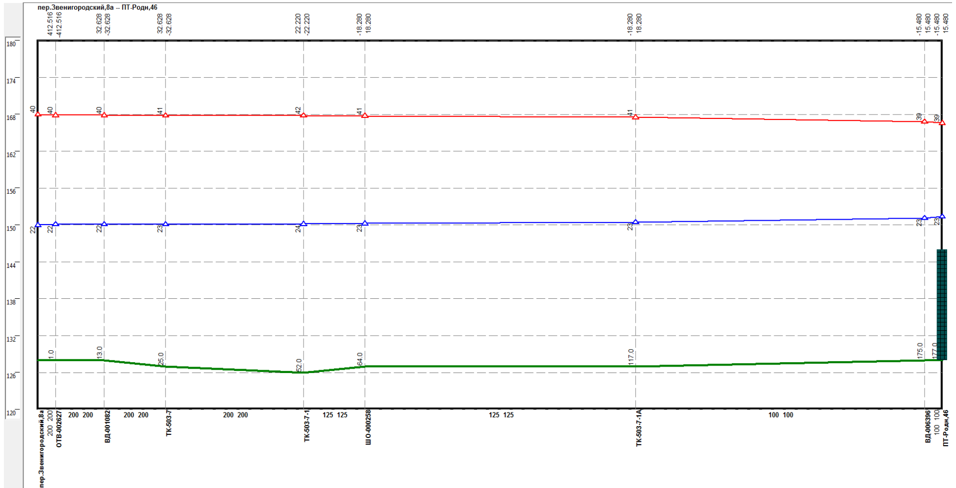
Рисунок 2.54 –Результат гидравлического расчета - график гидравлических режимов по пути теплоносителя от котельной пер. Звенигородский до ПТ-Родн,46
