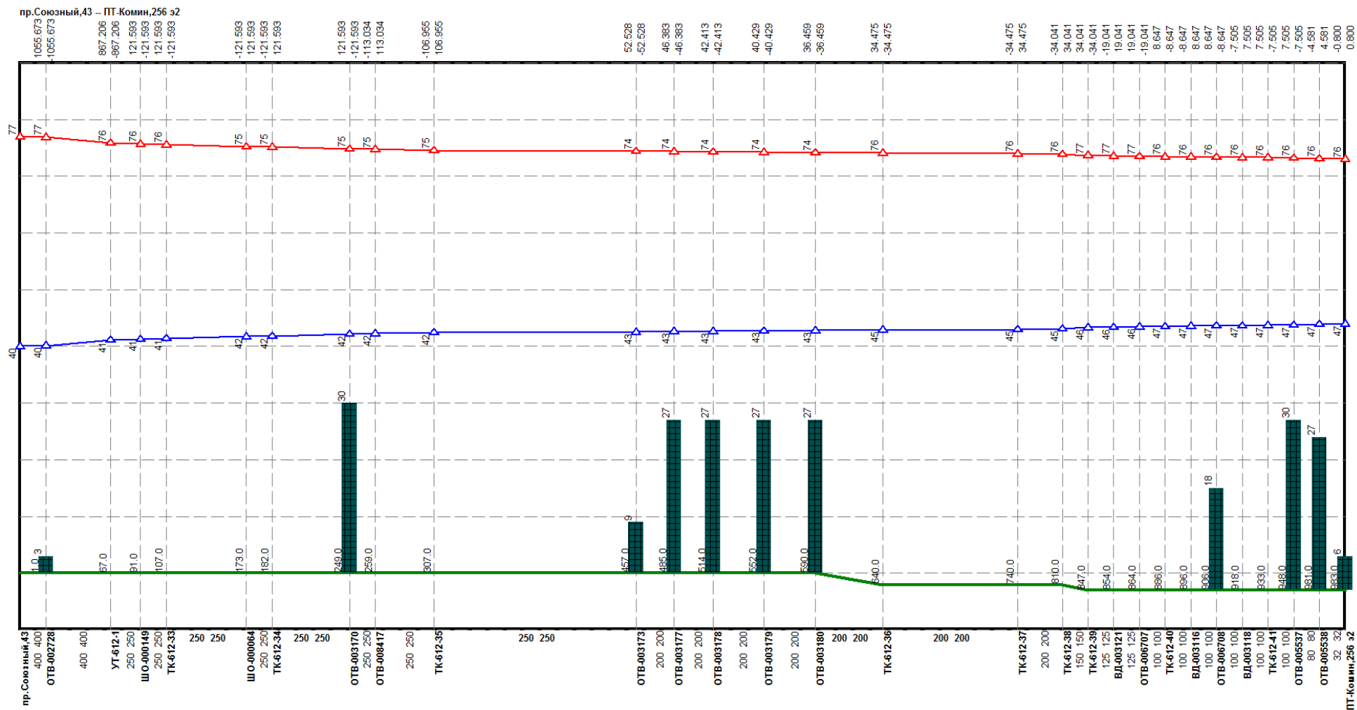
Рисунок 2.76 –Результат гидравлического расчета - график гидравлических режимов по пути теплоносителя от котельной пр. Союзный, 43 до ПТ-Комин, 256 э2
