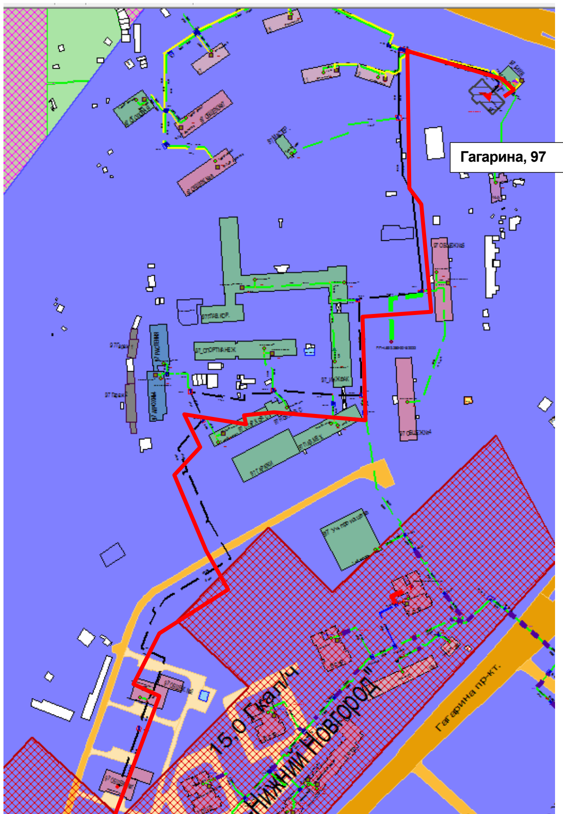
Рисунок 2.37 – Результат гидравлического расчета - расчетный путь теплоносителя от котельной пр. Гагарина, 97 до ПТ-Гагар,97 общ.№1
