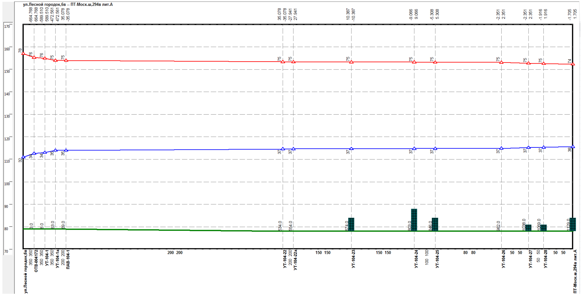
Рисунок 2.20 –Результат гидравлического расчета - график гидравлических режимов по пути теплоносителя от Лесной городок, 6в до ПТ-Моск.ш,294в лит.А
