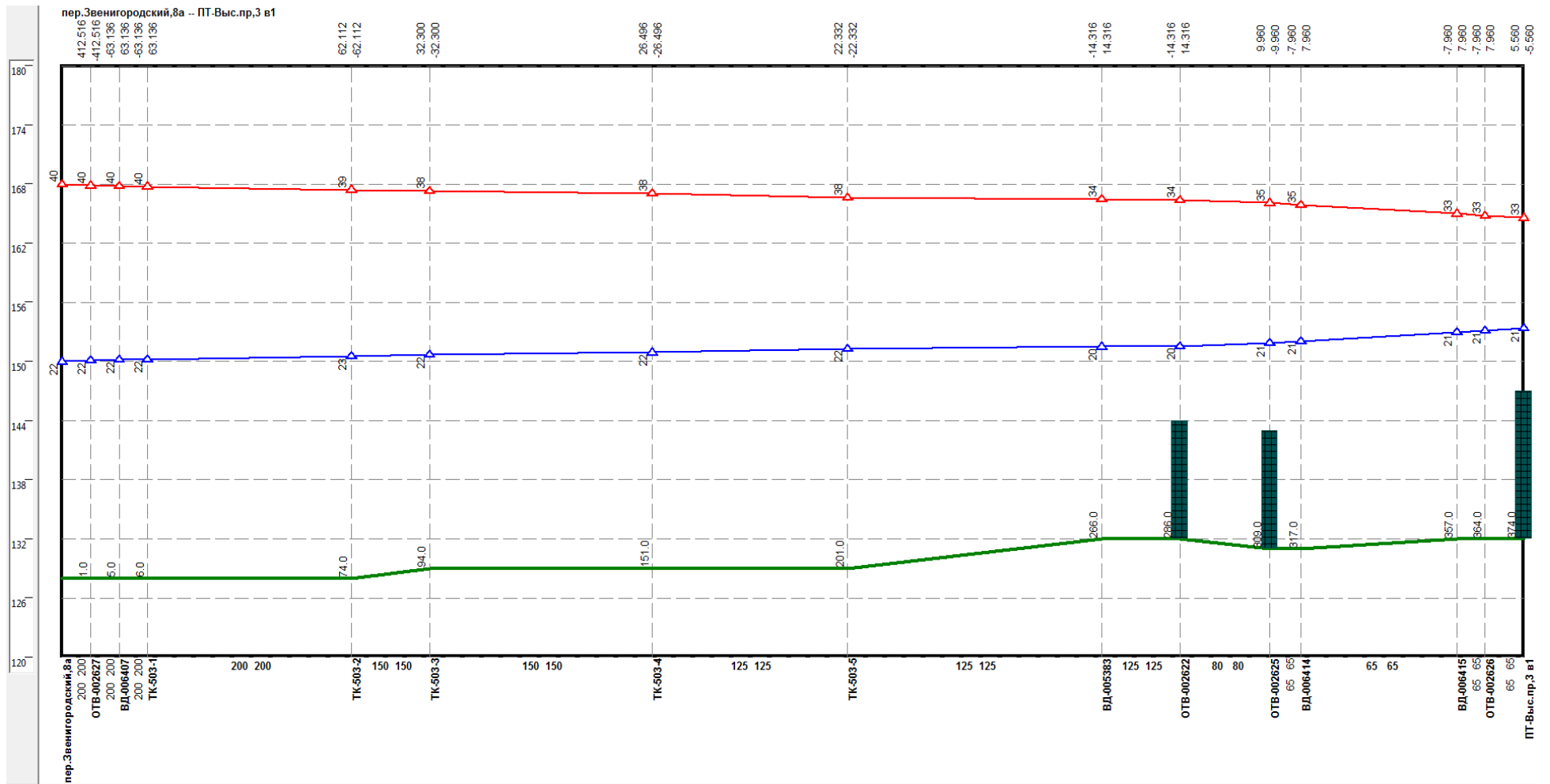
Рисунок 2.52 –Результат гидравлического расчета - график гидравлических режимов по пути теплоносителя от котельной пер. Звенигородский, 8а до ПТ-Выс.пр.3 в1
