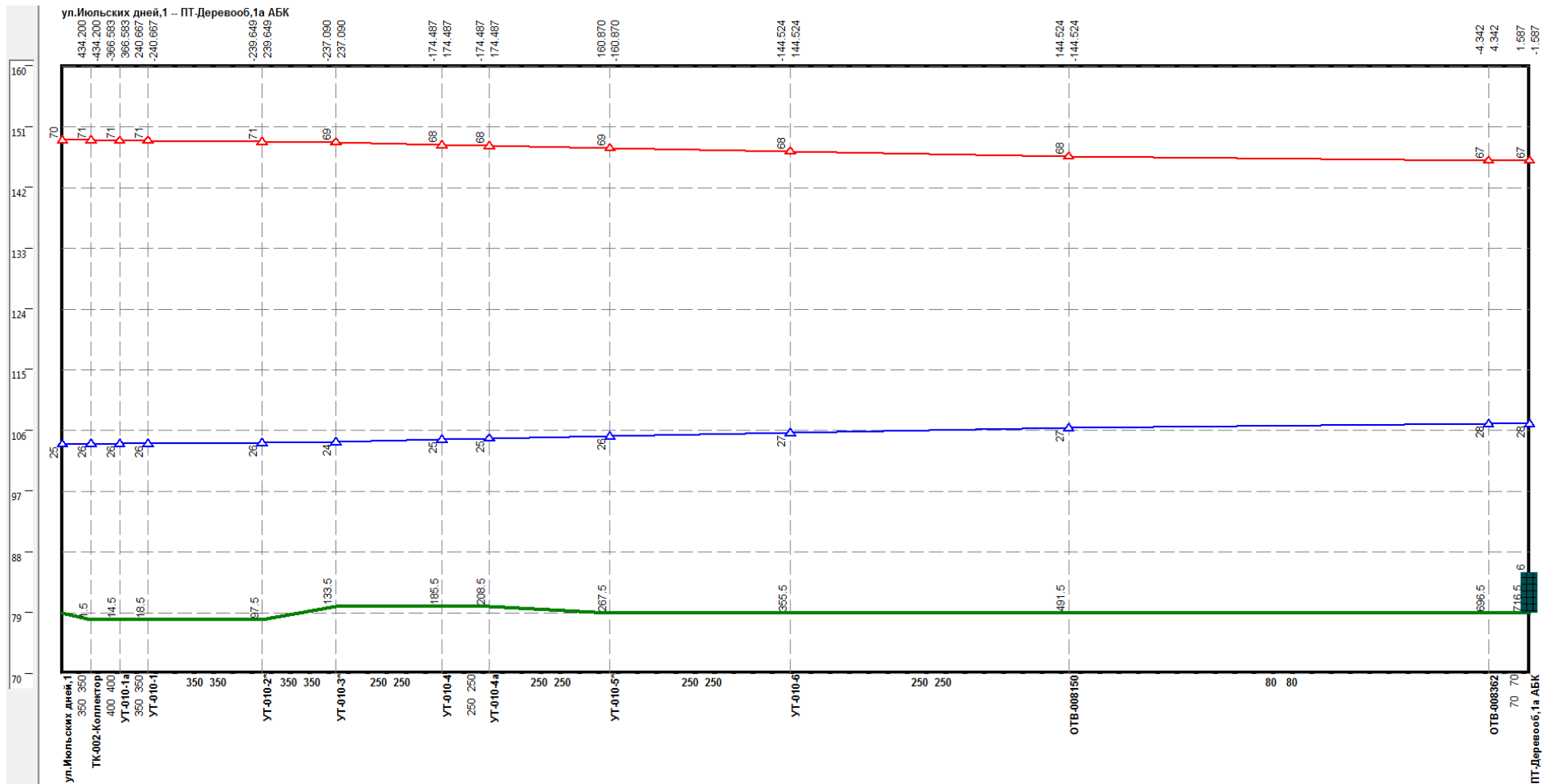
Рисунок 2.34 –Результат гидравлического расчета - график гидравлических режимов по пути теплоносителя от Июльских дней, 1 до ПТ-Деревооб, 1а АБК
