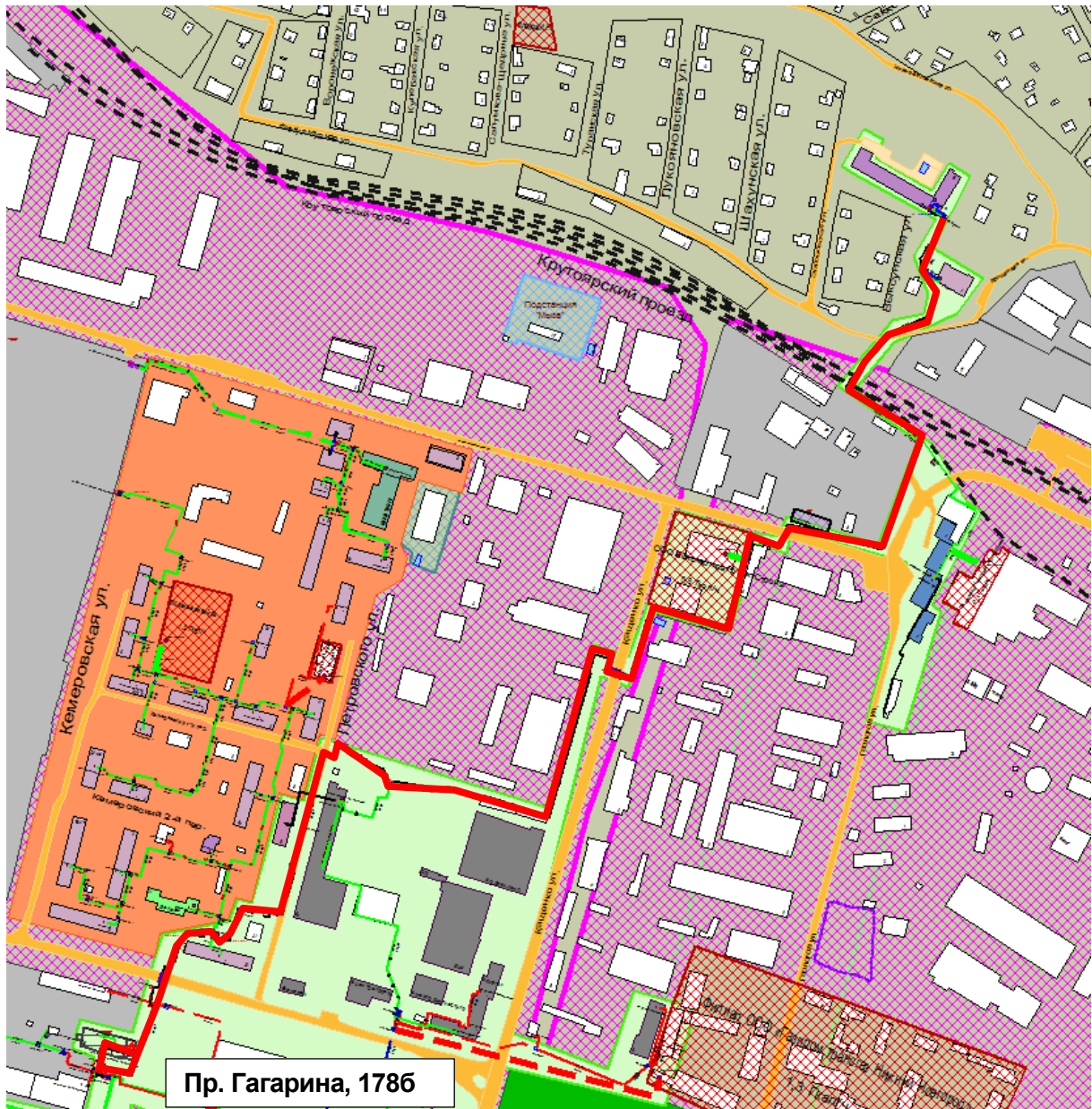
Рисунок 2.67 – Результат гидравлического расчета - расчетный путь теплоносителя от котельной пр. Гагарина, 1786 до ЦТП-706
