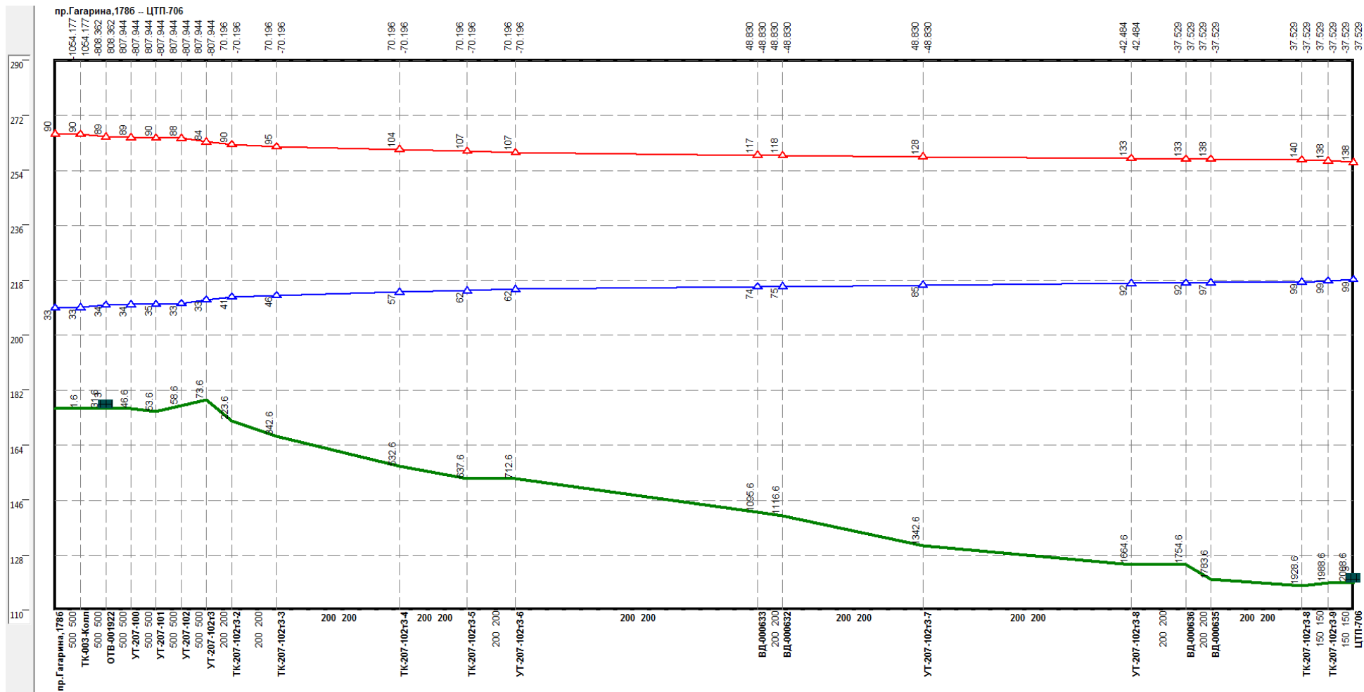
Рисунок 2.68 –Результат гидравлического расчета - график гидравлических режимов по пути теплоносителя от котельной пр. Гагарина, 1786 до ЦТП-706
