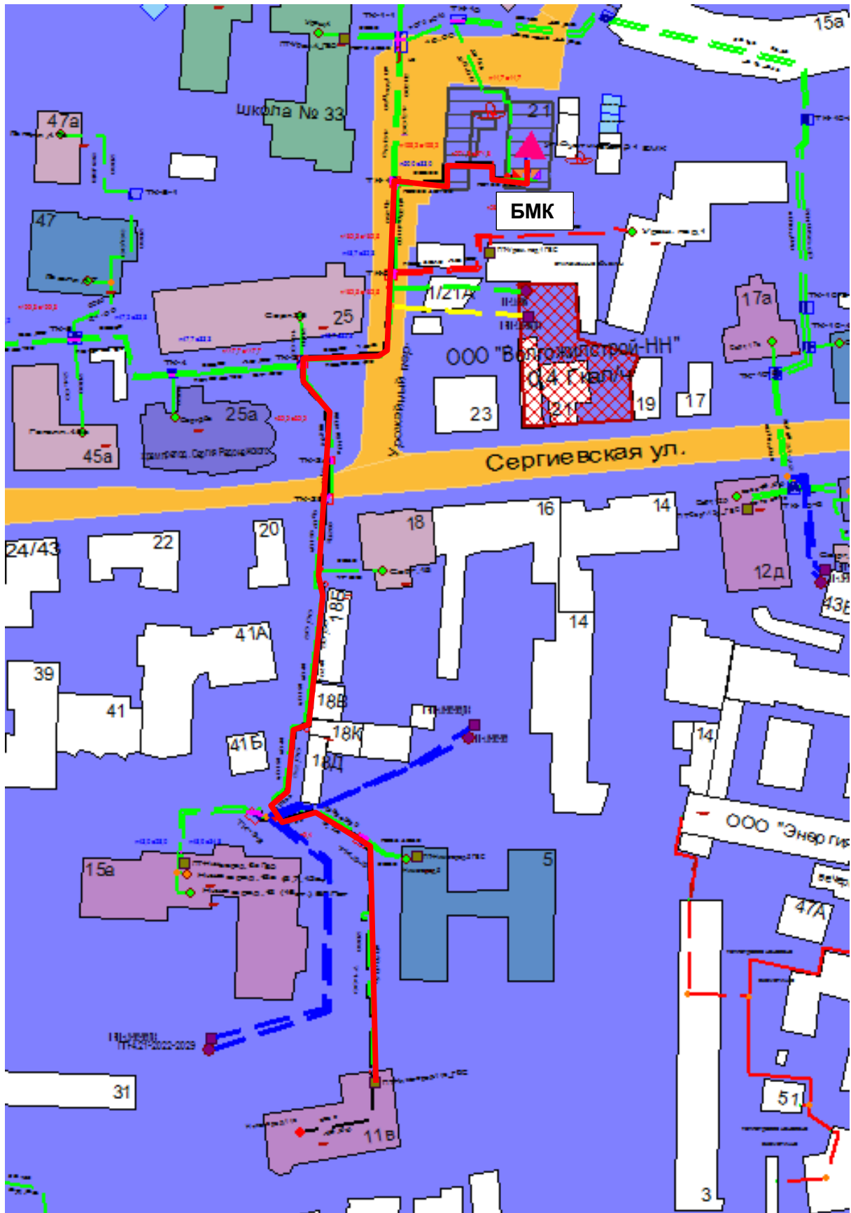
Рисунок 2.9 – Результат гидравлического расчета - расчетный путь теплоносителя от котельной Суетенская, 21 до ПТ-Нтжегород, 11в
