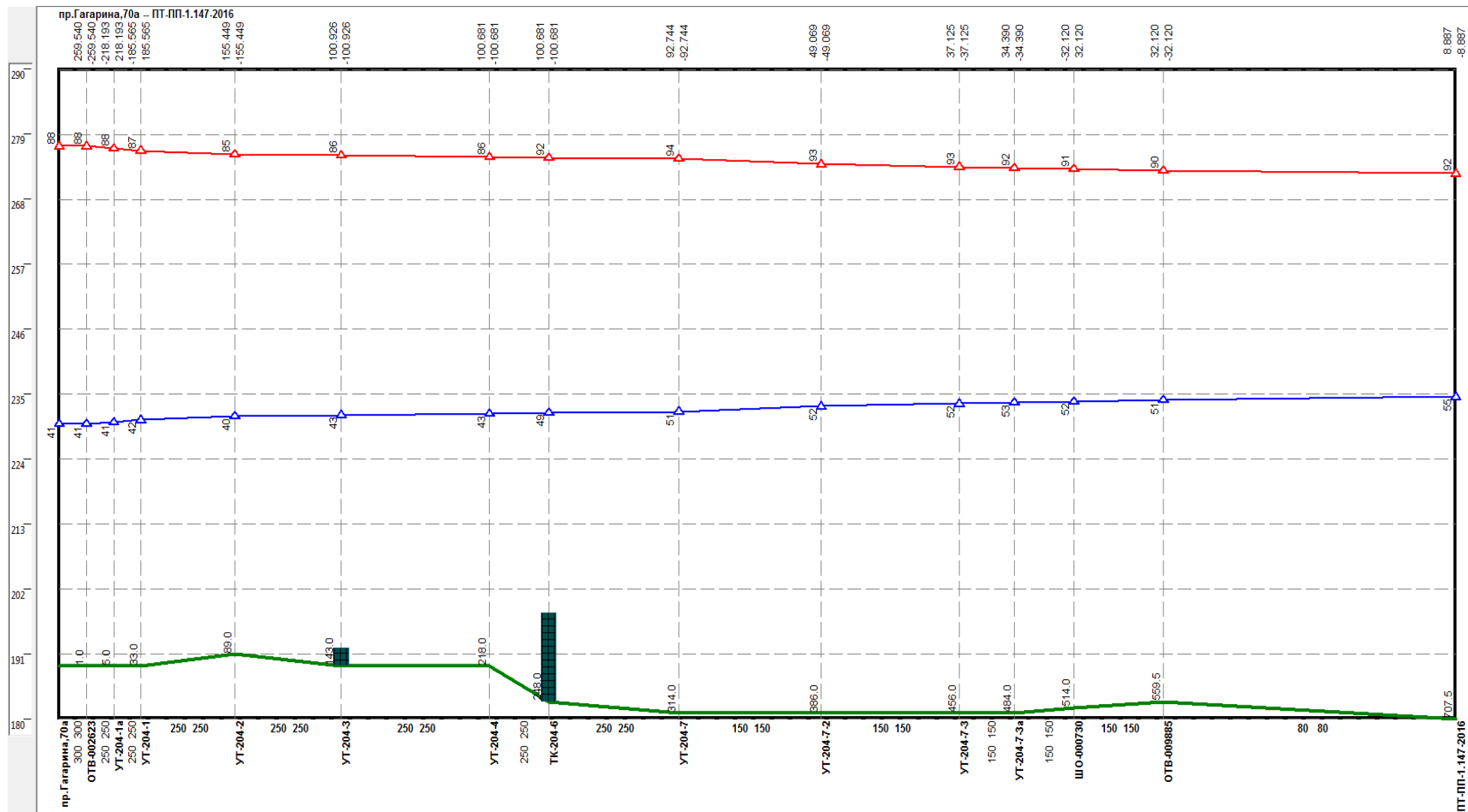
Рисунок 2.58 –Результат гидравлического расчета - график гидравлических режимов по пути теплоносителя от котельной пр. Гагарина, 70а до ПТ- ПП-1.147-2016.
