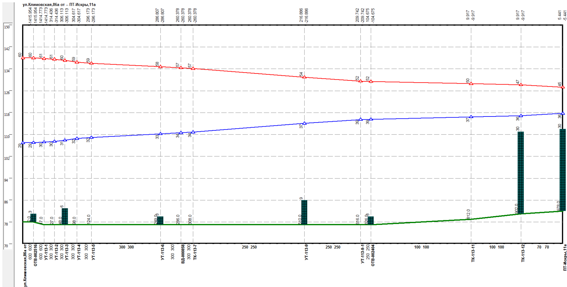
Рисунок 2.44 –Результат гидравлического расчета - график гидравлических режимов по пути теплоносителя от котельной Климовская, 86а до ПТ-Искры, 11а
