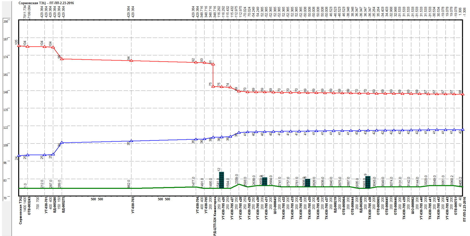
Рисунок 2.8 –Результат гидравлического расчета - график гидравлических режимов по пути теплоносителя от СТЭЦ до ПТ-ПП-2.23-2016
