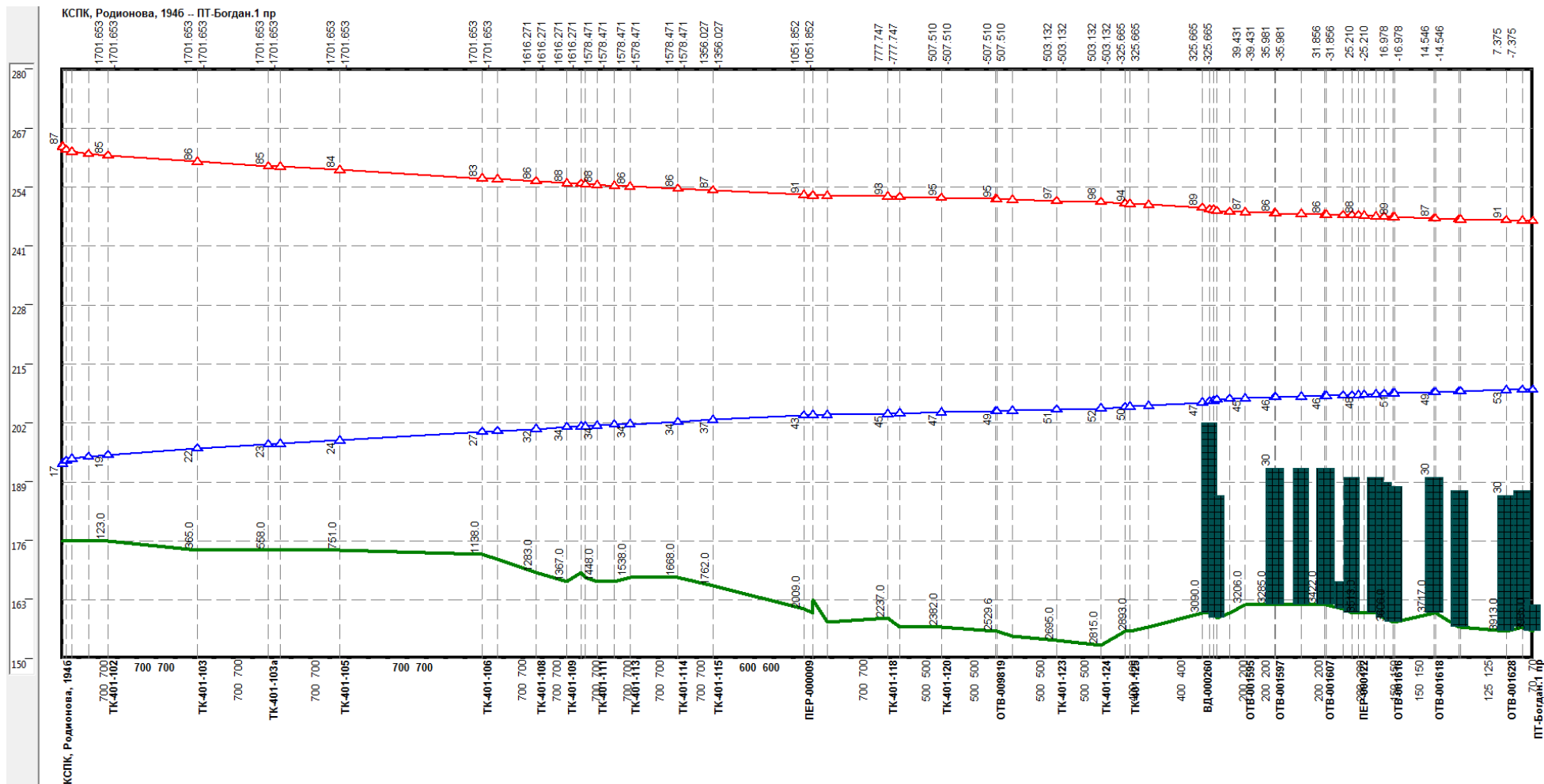
Рисунок 2.80 –Результат гидравлического расчета - график гидравлических режимов по пути теплоносителя от котельной ул. Родионова, 1946 до ПТ-Богдан, 1 пр.
