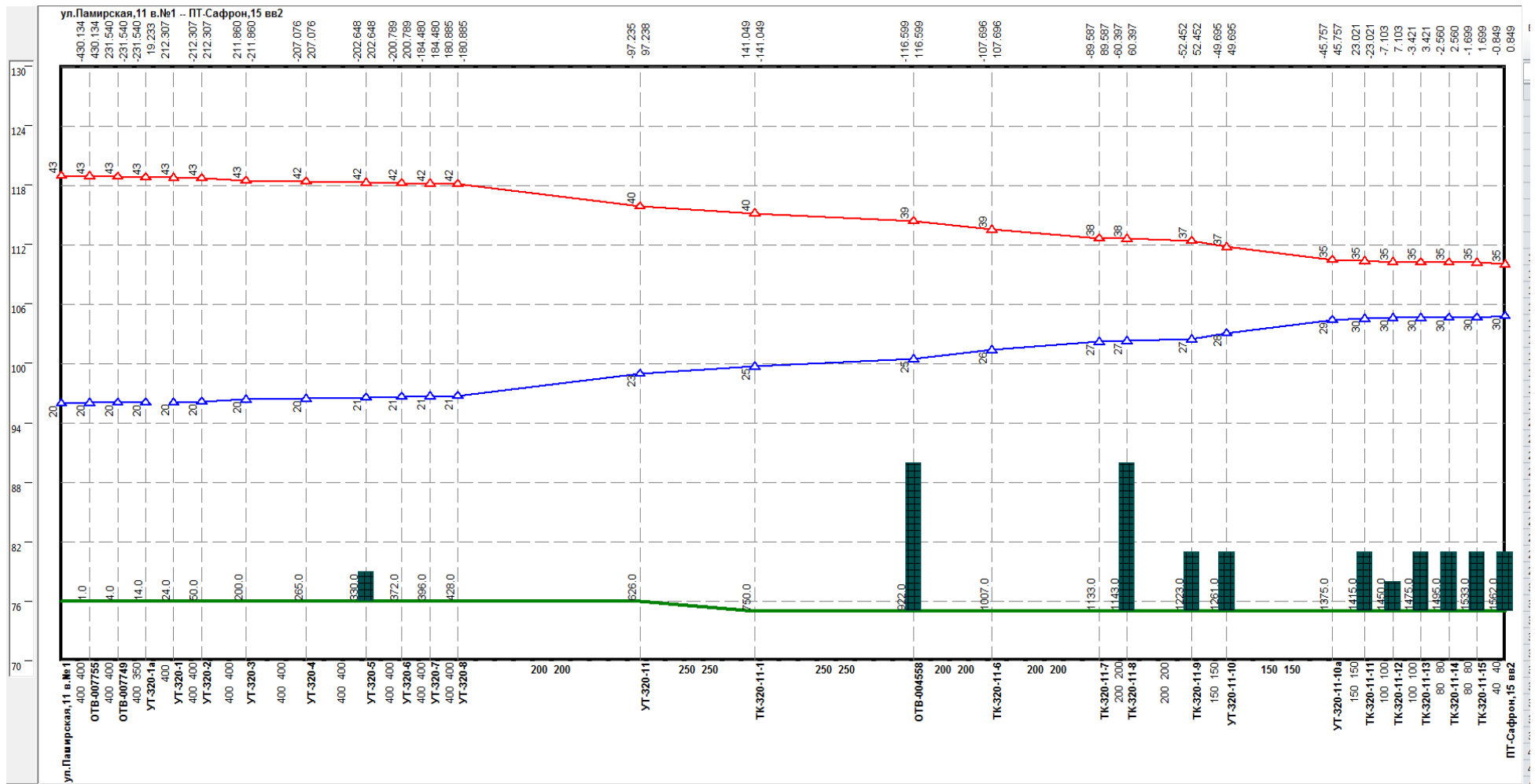
Рисунок 2.14 –Результат гидравлического расчета - график гидравлических режимов по пути теплоносителя от котельной Памирская, 11 до ПТ-Сафрон,15 вв2
