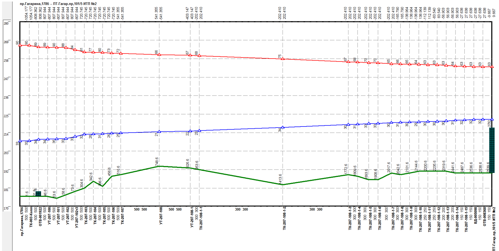
Рисунок 2.70 –Результат гидравлического расчета - график гидравлических режимов по пути теплоносителя от котельной пр. Гагарина, 1786 до ПТ-Гагар.пр.101/5 ИТП №2.
