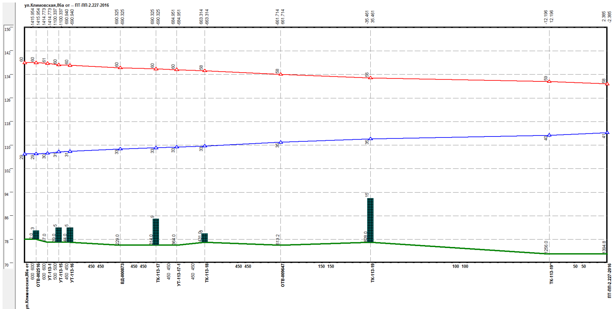
Рисунок 2.46 –Результат гидравлического расчета - график гидравлических режимов по пути теплоносителя от котельной Климовская, 86а до ПТ-ПП-2.227-2016
