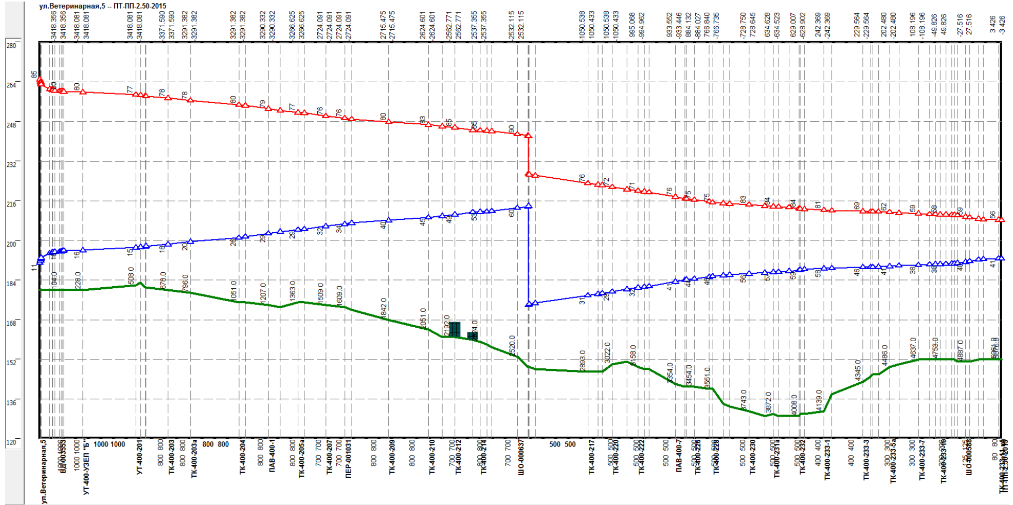
Рисунок 2.62 –Результат гидравлического расчета - график гидравлических режимов по пути теплоносителя от котельной НТЦ до ПТ- ПП-2-50-2015.
