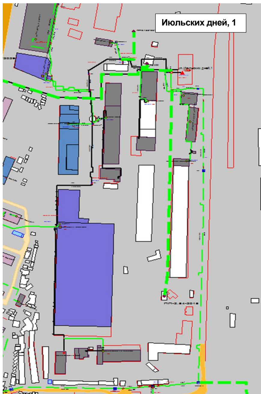
Рисунок 2.33 – Результат гидравлического расчета - расчетный путь теплоносителя от Июльских дней, 1 до ПТ-Деревооб, 1а АБК
