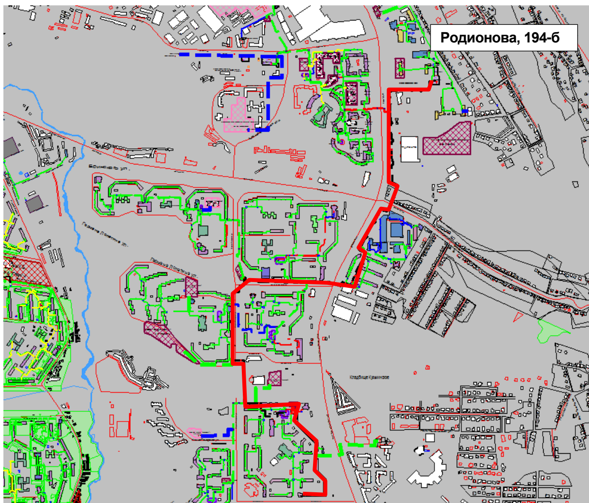
Рисунок 2.79 – Результат гидравлического расчета - расчетный путь теплоносителя от котельной ул. Родионова, 1946 до ПТ-Богдан, 1 пр.
