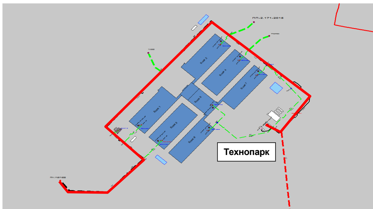
Рисунок 2.35 – Результат гидравлического расчета - расчетный путь теплоносителя от котельной «ТЕХНОПАРК» до ПТ-ПП-1,17-2017-2022.
