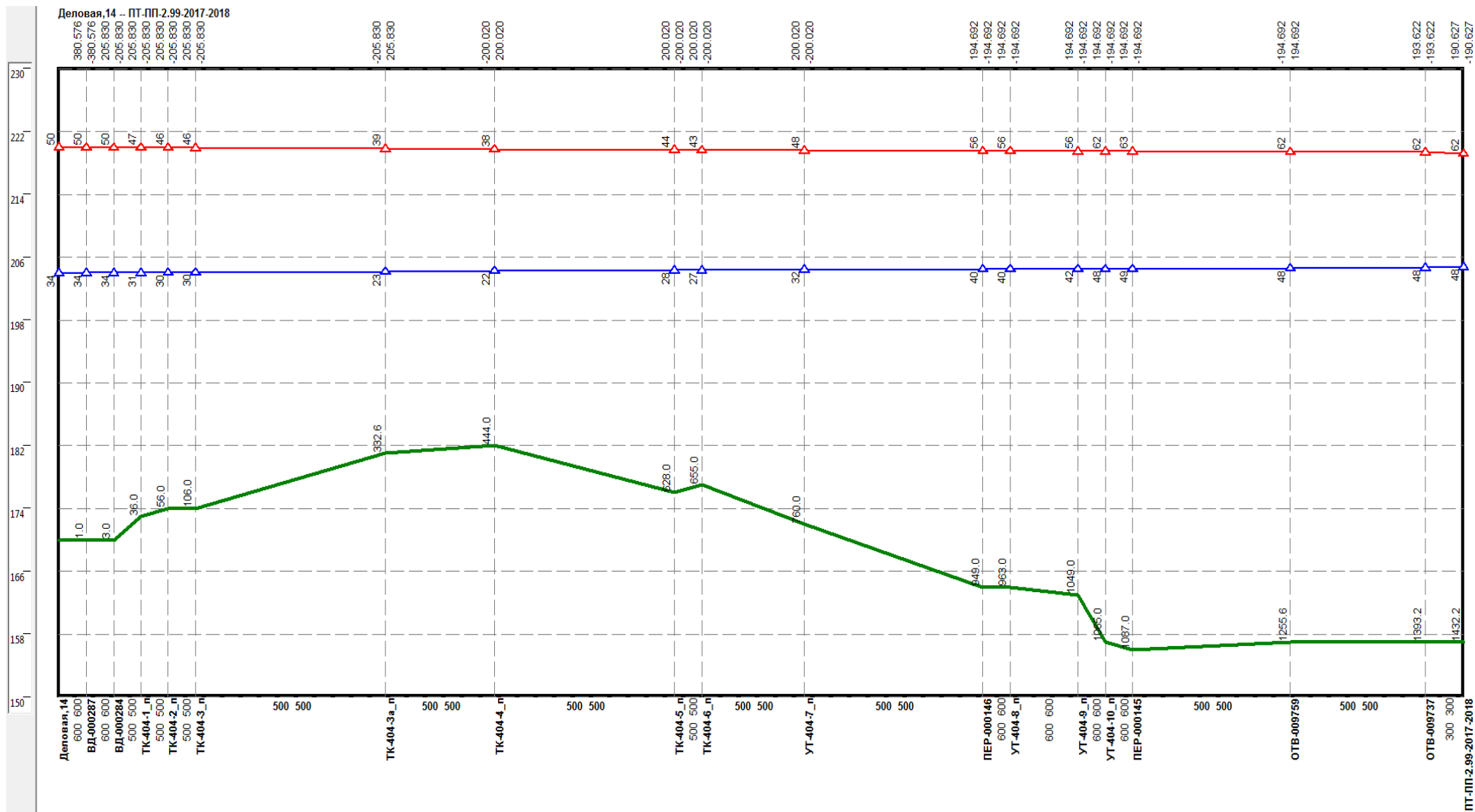
Рисунок 2.30 –Результат гидравлического расчета - график гидравлических режимов по пути теплоносителя от котельной Деловая, 14 до ПТ-ПП-2.99-2017-2018.
