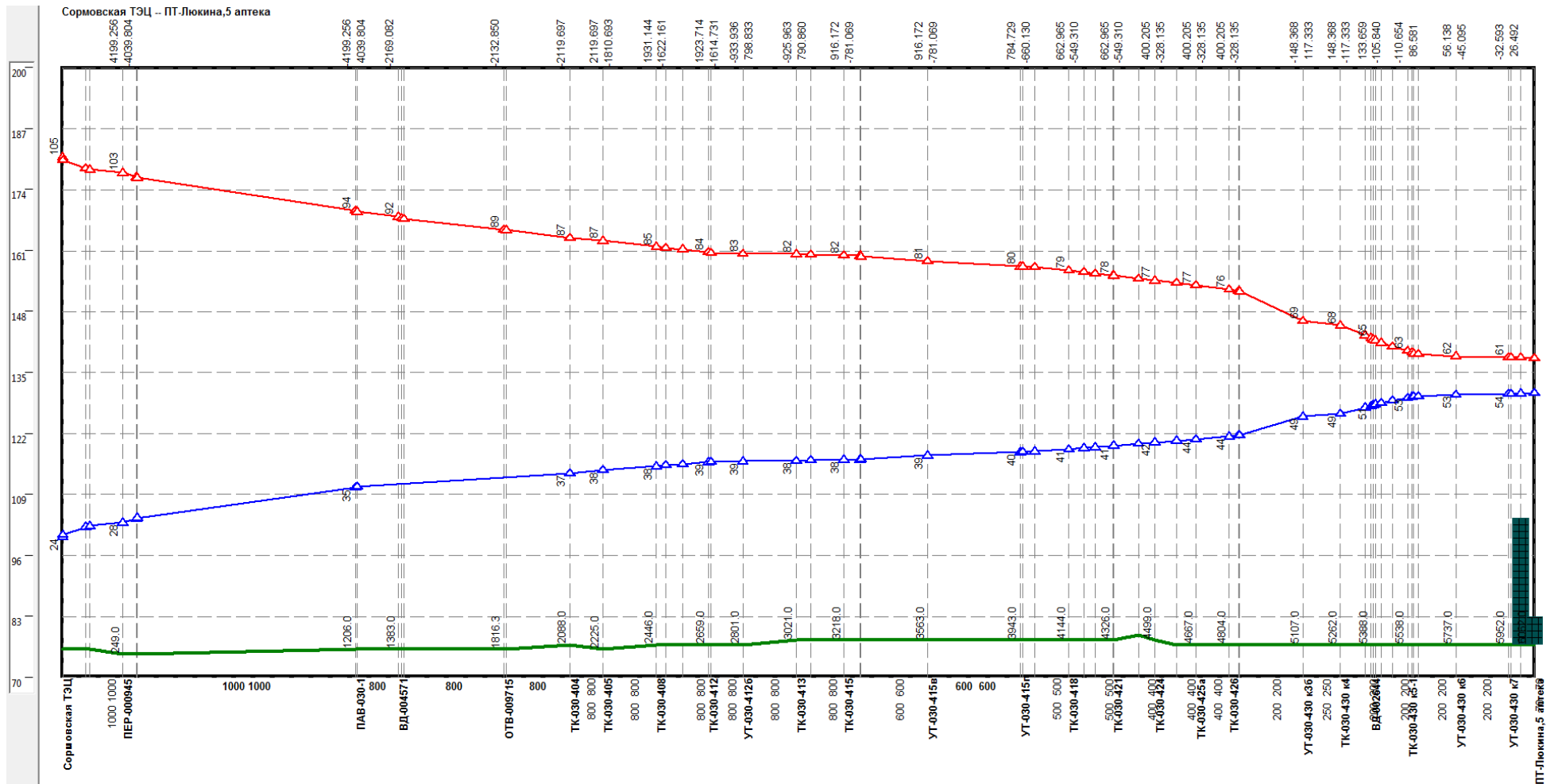
Рисунок 2.2 –Результат гидравлического расчета - график гидравлических режимов по пути теплоносителя от СТЭЦ до ПТ-Люкина,5 аптека
