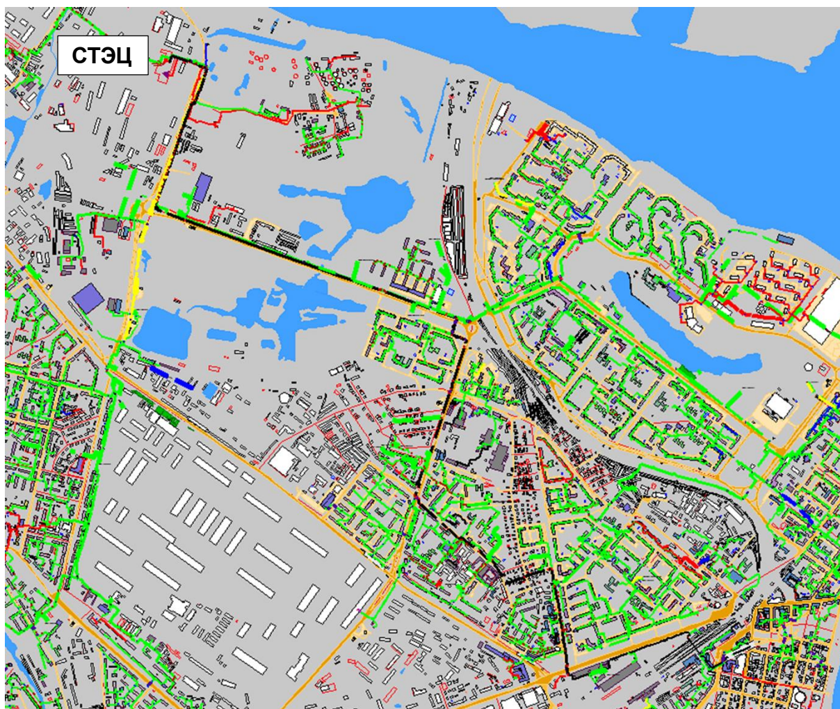
Рисунок 2.5 - Результат гидравлического расчета - расчетный путь теплоносителя от СТЭЦ до ПТ-Сорм.ш,20 э2
