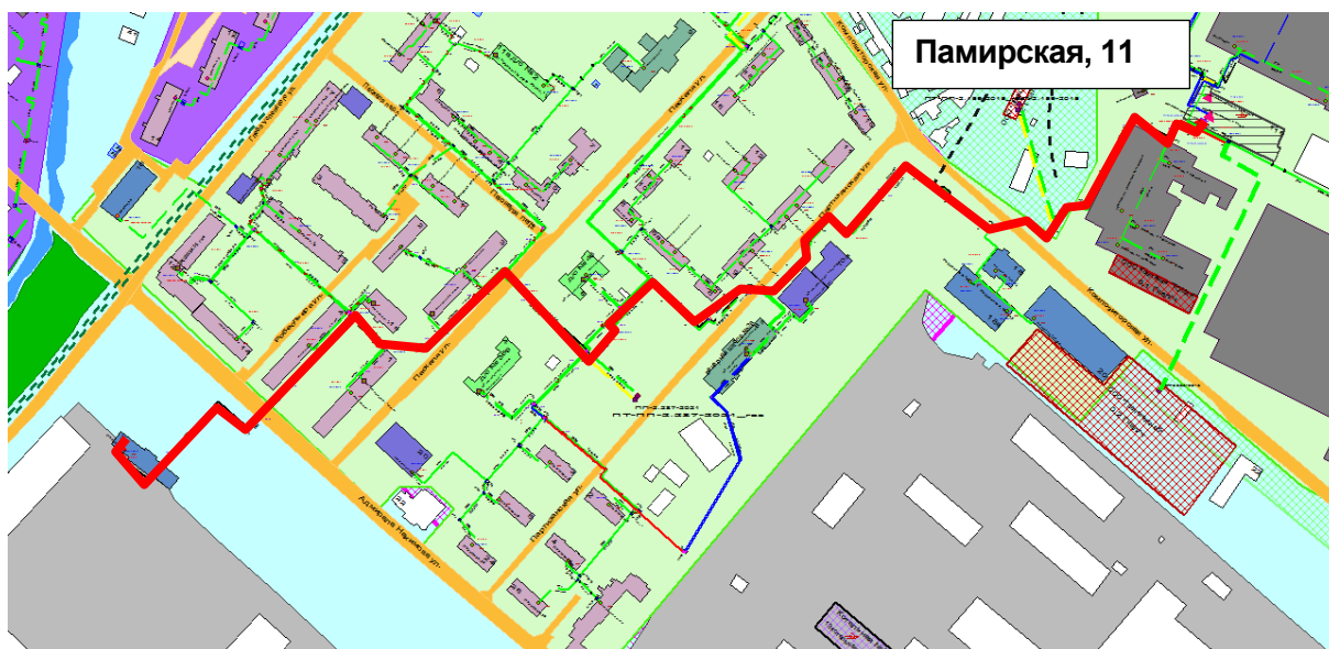
Рисунок 2.15 – Результат гидравлического расчета - расчетный путь теплоносителя от котельнио Памирская, 11 до ПТ-Нахимова,3
