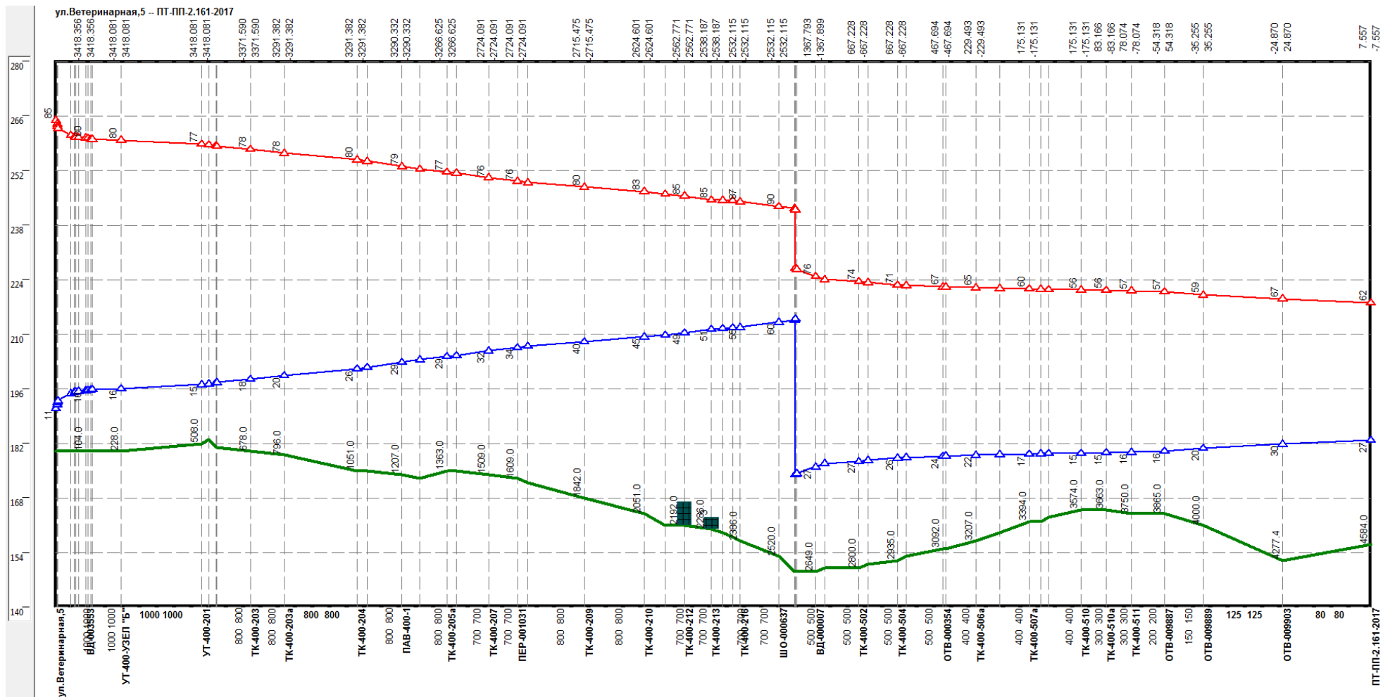
Рисунок 2.64 – Результат гидравлического расчета - график гидравлических режимов по пути теплоносителя от котельной НТЦ до ОТВ-009903
