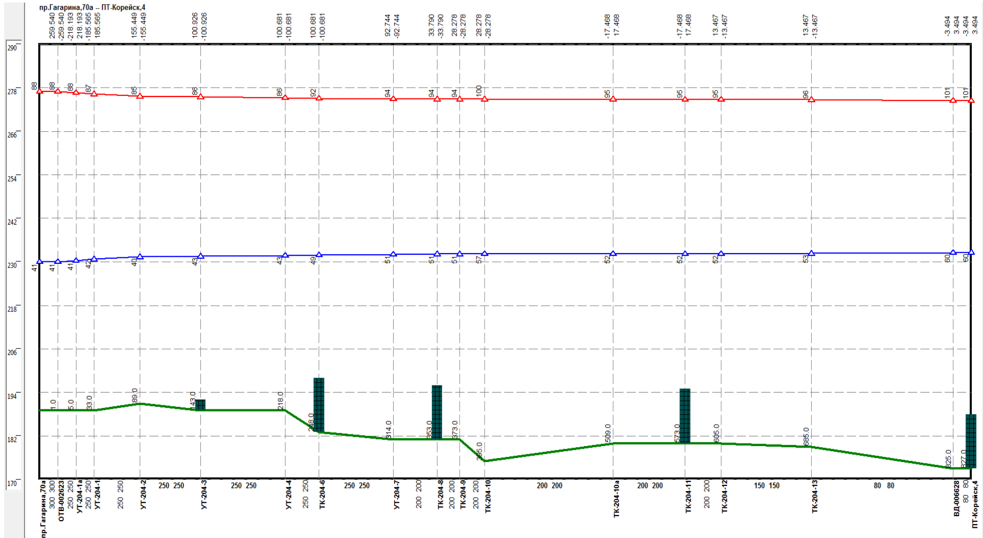
Рисунок 2.56 –Результат гидравлического расчета - график гидравлических режимов по пути теплоносителя от котельной пр. Гагарина, 70а до ПТ-Корейск, 4
